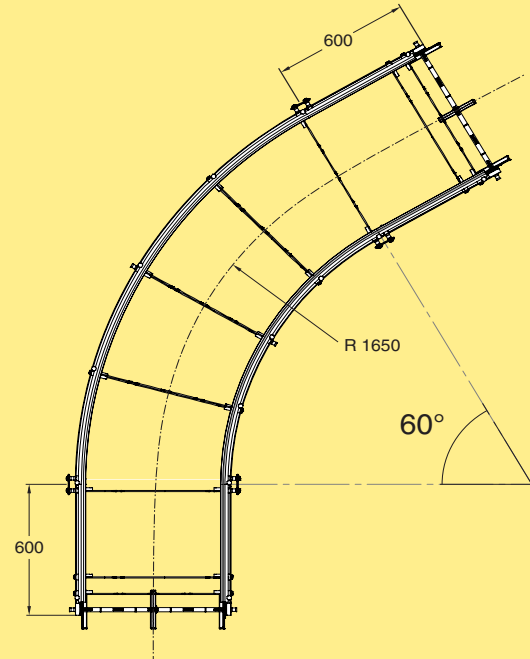
Plain bend, 60°±1° R=1650±10 mm
