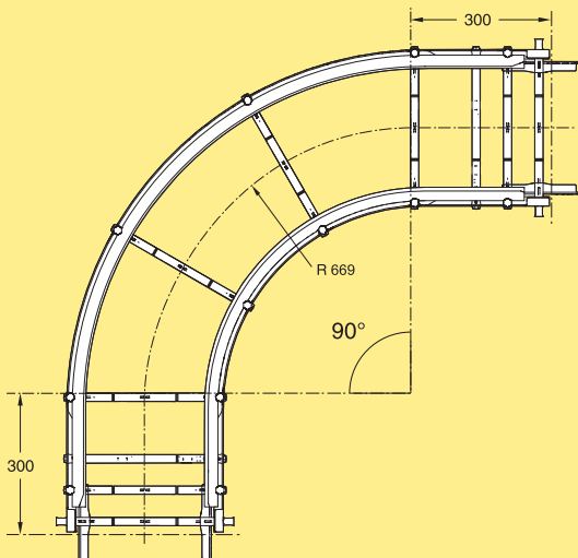
Gleitbogen, 90°±1° R=669±10 mm WLBPX 90A374 S
