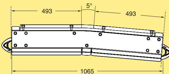
Vertikaler Gleitbogen, 5°, neg. WLBVX 5A374N
