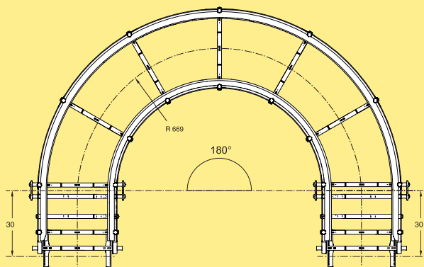
Gleitbogen, 180°±1° R=669±10 mm WLBPX 180A374 S
