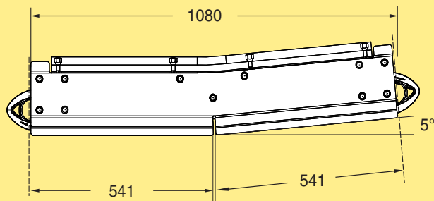
Vertikaler Gleitbogen, 5°, pos. WLBVX 5A374P
