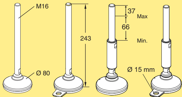
Stellfuß M16 M16, Verankerung M16, EHEDG/3A M16, EHEDG/3A, Befestigung XCFCX 16x80 A XCFCX 16x80 H XCFCX 16x80 HA
