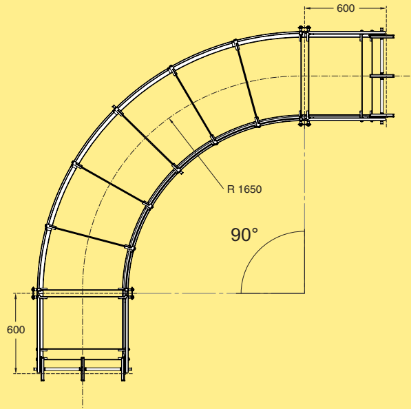
Plain bend, 90°±1° R=1650±10 mm WLBPX 90A678
